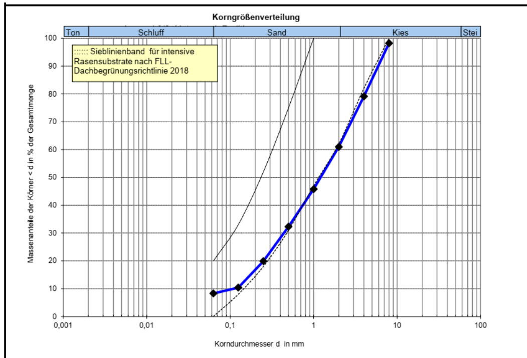
Abbildung 1: Körnungssummenlinie (Sieblinie des untersuchten Substrats), eingezeichnet ins Sieblinienband für Mehrschicht-Rasensubstrate nach FLL-Dachbegrünungsrichtlinie 2018
